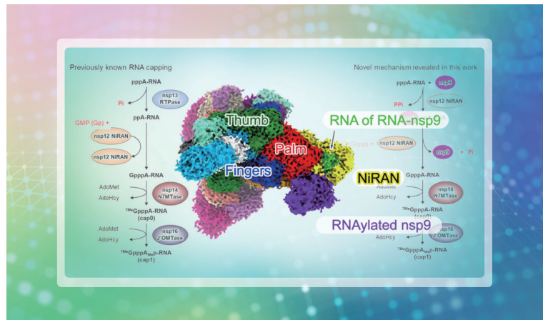
新冠病毒转录复制复合体。
