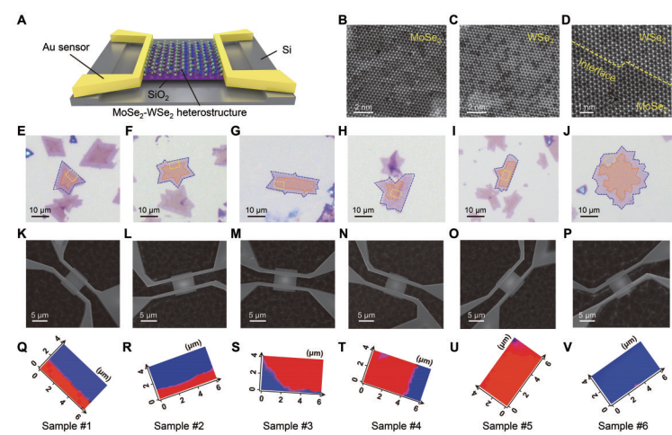
不同界面角度MoSe 2 -WSe 2 异质结器件的制备与表征。
